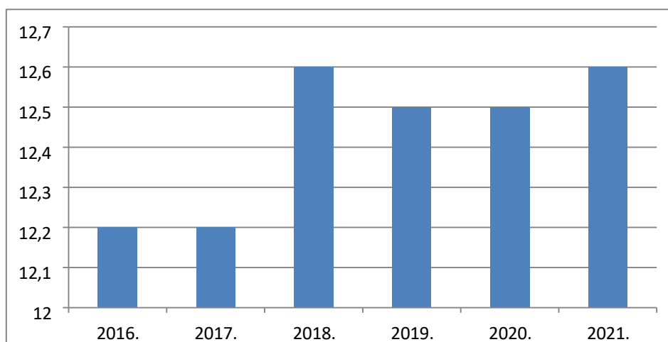
Дијаграм 2. Средња годишња температура на мјерној станци Добој за период 2016-2021.
