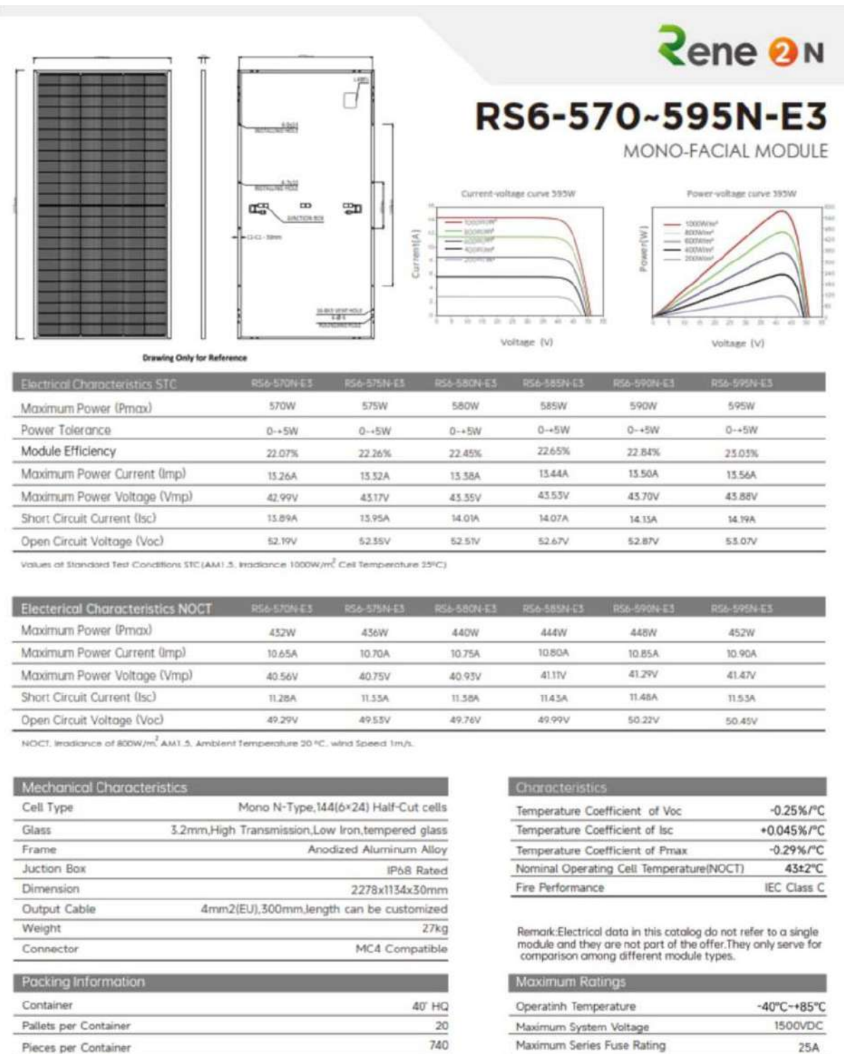
Slika br.11 Karakteristike solarnog panela
