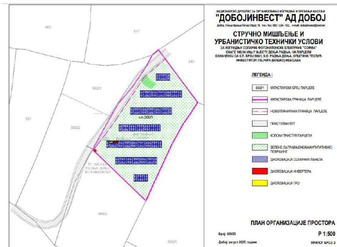
Slika br. 2. plan organizacije prostora
